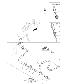
ETB-000931, Zespół do rozszewu granicznego, limiter M --- hydraulika
