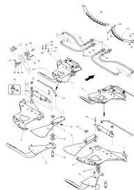
ETB-000937, Dno z otworami mechaniczne
