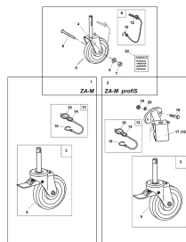
ETB-000968, Urządzenie transportowe i postojowe
