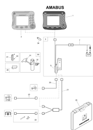
ETB-000955, AMABUS AMATRON 3 do rocznika model. 2020 włącznie
