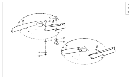
ETB-000925, Podstawowe łopatki rozszewniające
