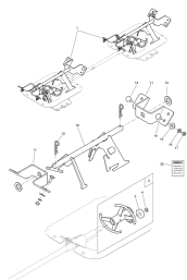
ETB-000936, Mieszadło mimośrodowe
