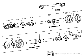
ETB-0000005724, Wałek przegubowo-teleskopowy EJ685 - SD05, 810 mm, z widelcem Russia
