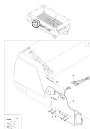
ETB-0000009698, Uchwyt ze śrubą przegubową do AmaTron+
