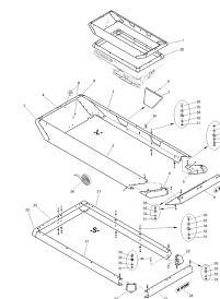
ETB-000950, Nadstawka L 1000 / S 500
