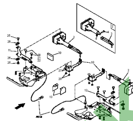
ETB-000938, Dno z otworami elektryczne
