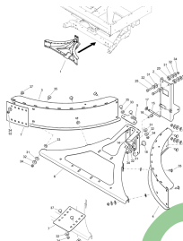
ETB-000972, Ekran krawędziowego jednostronny sterowany ręcznie
