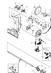
ETB-000935, Wałek mieszadła z jarzmem łańcucha
