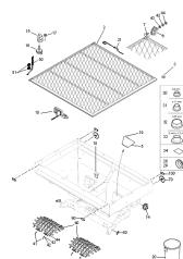
ETB-000916, Rama i zbiornik --- sito / korki / kratka ochronna mieszadła
