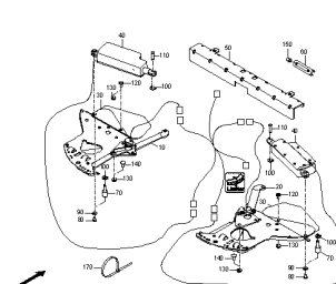
ETB-0000002874, Pakiet elektroniki Easy 2
