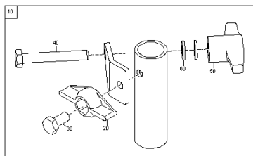
ETB-0000009698, Uchwyt ze śrubą przegubową do AmaTron+
