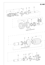
ETB-000965, Wałek przekątnikowy W2102, 760 mm EJ448
