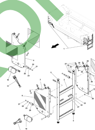
ETB-000961, Oświetlenie przednie i drabina do nadstawki L1000
