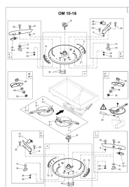
ETB-000920, Tarcza rozsiewająca OM 10-16
