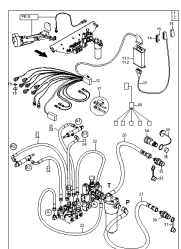
ETB-000944, Pakiet elektroniki Comfort ZA-M Ultra/Profis od 03.2010!
