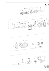
ETB-000966, Wałek przekątnikowy WTS100E Tele-Space, 810 mm EJ451
