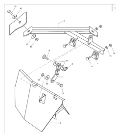
ETB-000929, Osłona do rozszewu granicznego
