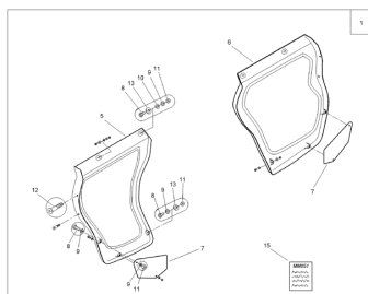
ETB-000971, Osłona przeciwbłotna, zestaw bezpieczeństwa
