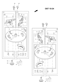
ETB-000924, Tarcza rozszewniająca OST 10-24
