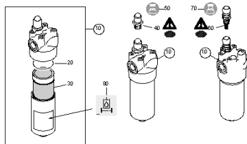
ETB-006791, Filtr hydrauliczny ciśnieniowy
