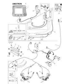
ETB-000954, AMATRON+ do rocznika model. 2020 włącznie
