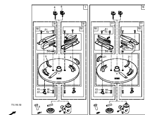
ETB-000928, Tarcza do rozszewu granicznego TS 15-18
