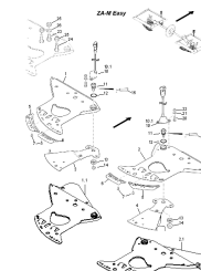
ETB-000939, Dno z otworami EasySet / Easy 2
