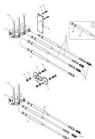
ETB-000948, Zespół dwudrogowy
