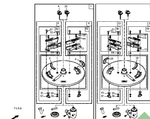
ETB-000926, Tarcza do rozszewu granicznego TS 5-9
