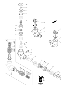
ETB-000934, Przekładnia kątowna
