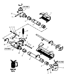
ETB-000932, Napęd ZA-M
