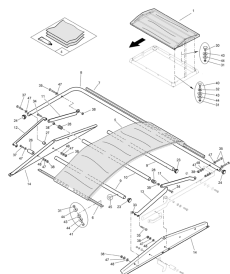
ETB-000951, Składana plandeka
