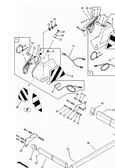
ETB-000962, Zestaw bezpieczeństwa
